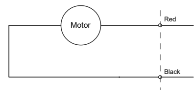
Motor wiring
